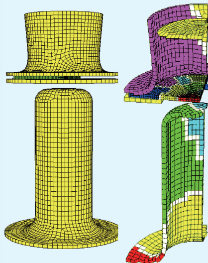
金型のプレス加工並列接触解析
