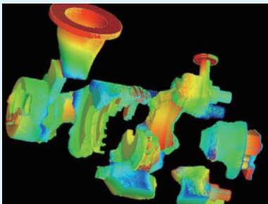
領域分割による並列計算 (1億自由度ポンプモデルの応力解析)
