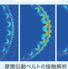
摩擦伝動ベルトの接触解析
