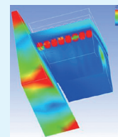
レール・車輪間の転がり接触解析
