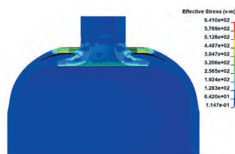
高圧水素容器の衝撃損傷解析
