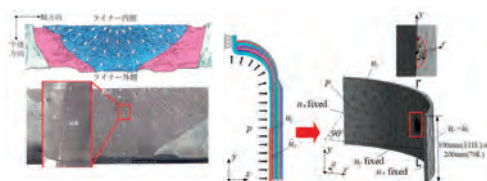
ズーム解析による超高圧複合圧力容器蓄圧器の疲労き裂進展寿命予測
