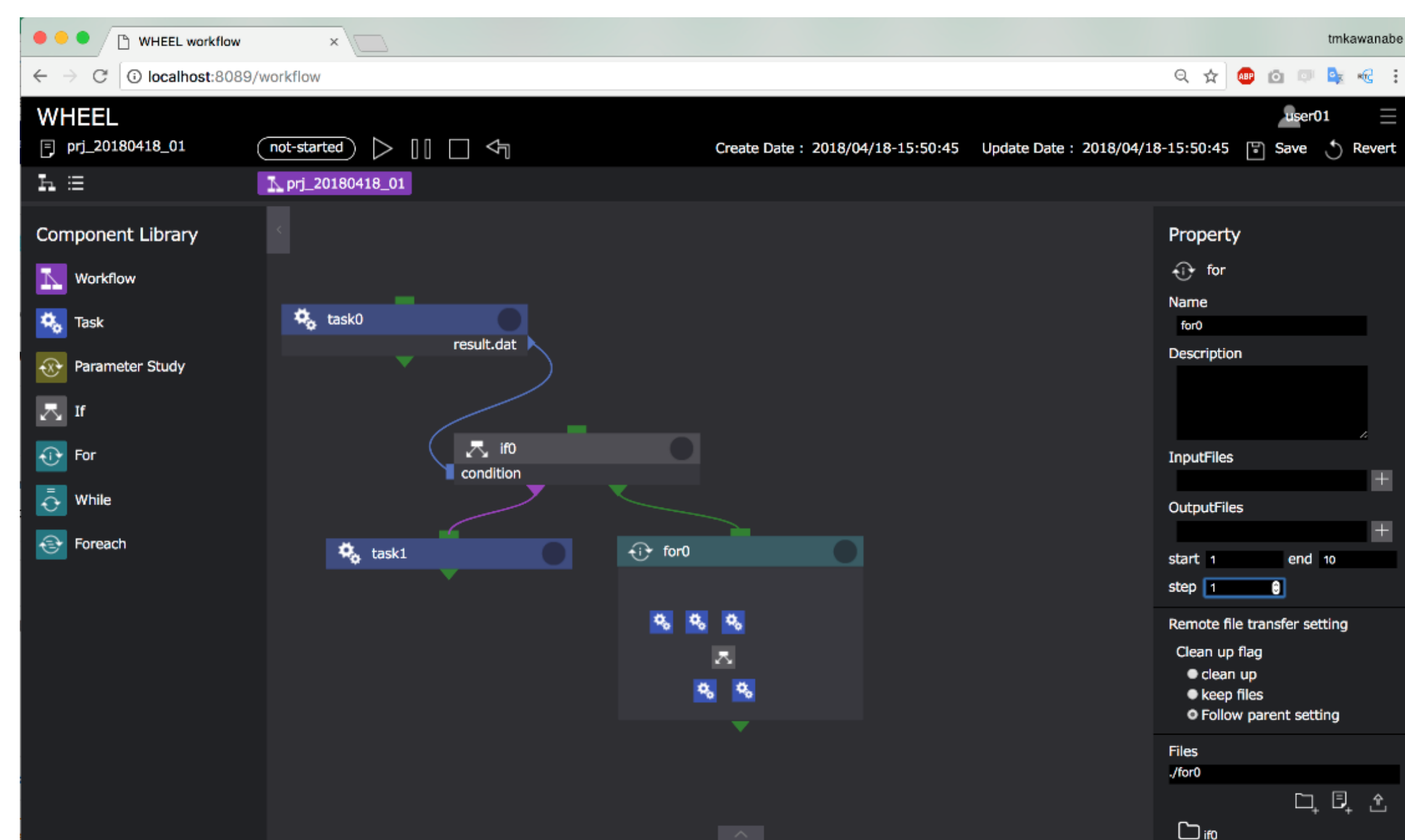
Webベースのワークフローシステム WHEEL
