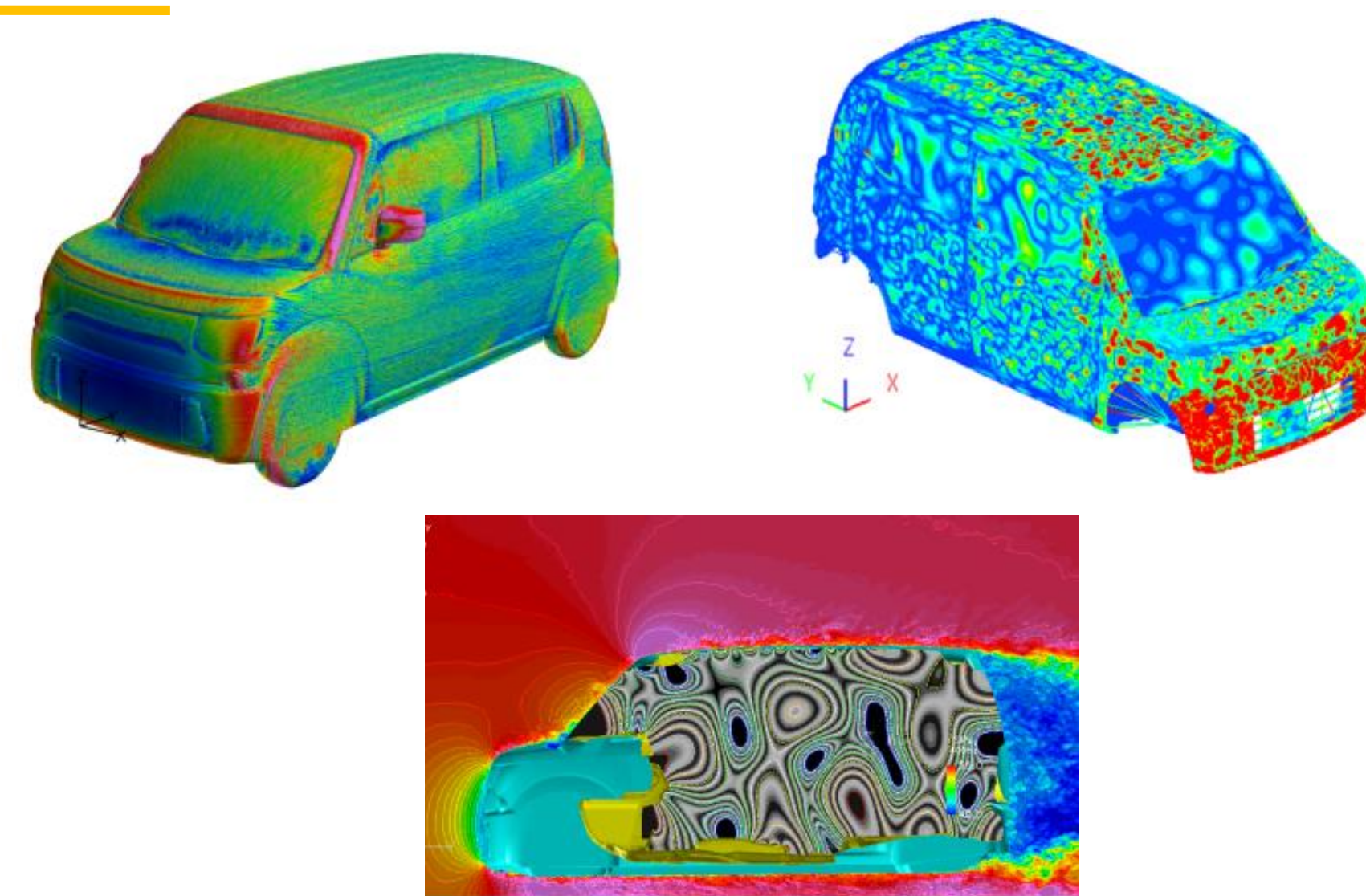
車内騒音予測システムの概要(流体・構造 振動・音響連成解析) ＜共同研究：豊橋技術科学大学, スズキ株式会社＞
